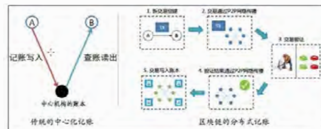
图 3 区块链式记账
